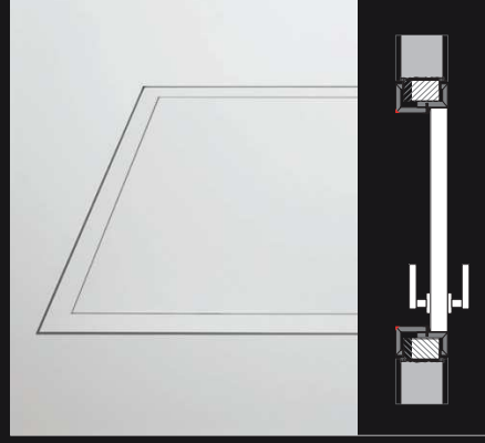
CUBE® Element Flächenverbund Tür | Zarge und Wand Blindstock mit Alu-Putzkante wird vor dem Verputzen in die Wand montiert
